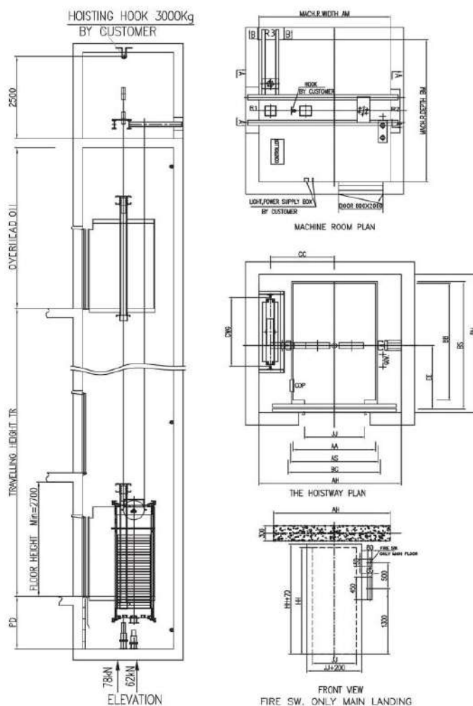
YS-MMR Mini MR bed elevator (center opening)
